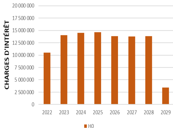
STRATEGIE H0
