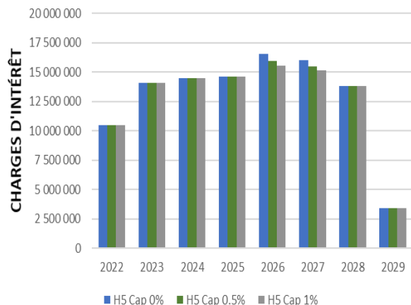
STRATEGIE H5
