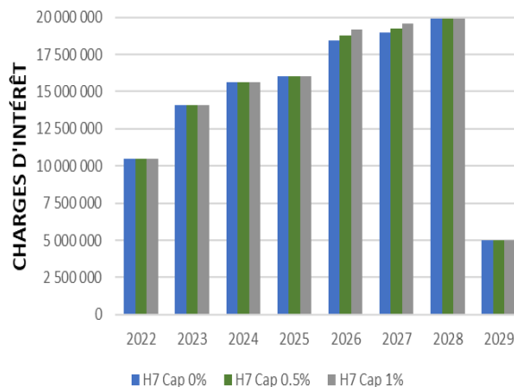
STRATEGIE H7
