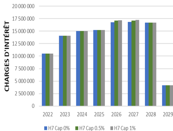
STRATEGIE H7
