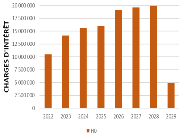
STRATEGIE H0
