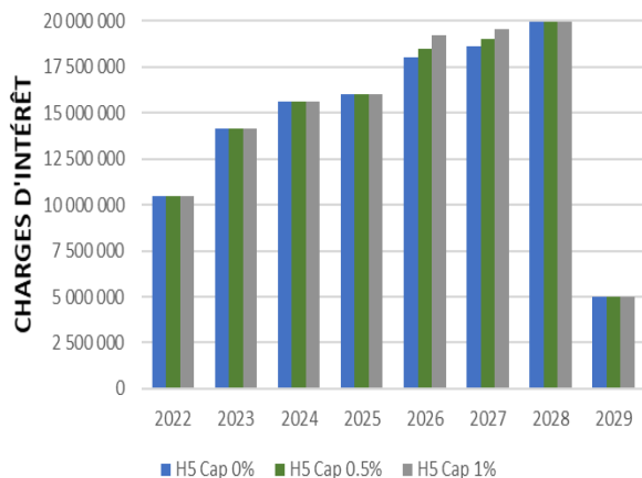
STRATEGIE H5
