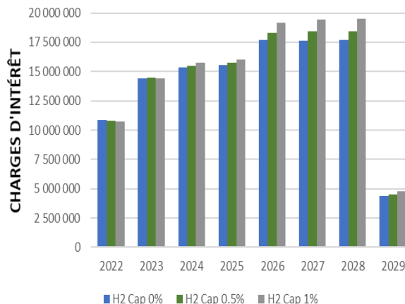
STRATEGIE H2
