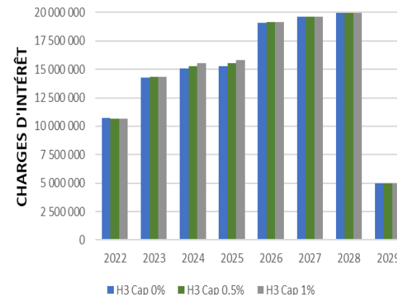
STRATEGIE H3
